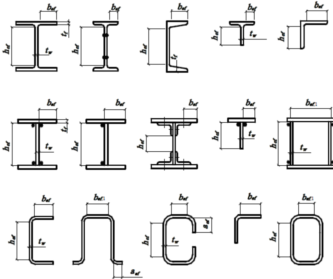
Рисунок 5 - Расчетные размеры стенок, свесов полок, поясных листов в прокатных, составных и гнутых профилях полную высоту стенки - в сварных элементах;
