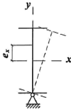
Рисунок Д.1 - Схема сечения элемента, подкрепленного вдоль полки Коэффициент \alpha следует определять по формуле (Ж.4) приложения Ж.
