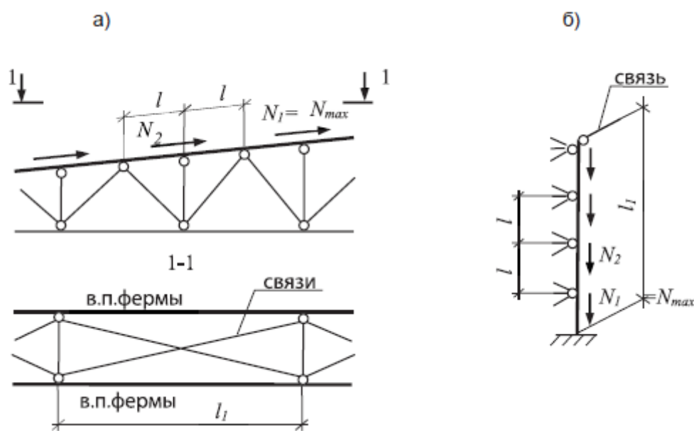
а) - пояса фермы; б) - ветви колонны
