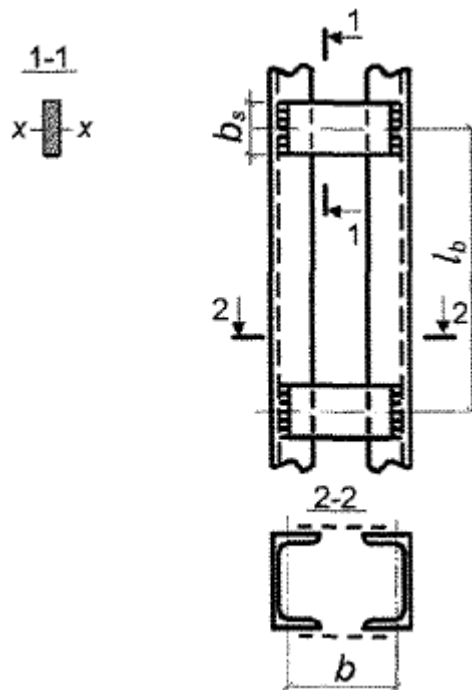
Рисунок 4* - Сквозной стержень с планками
